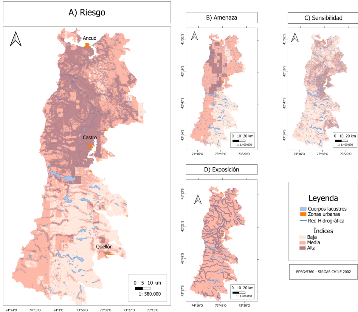
Figura 4. Índice de riesgo de los servicios ecosistémicos de provisión y regulación de agua dulce en la isla grande de Chiloé. (A) índice de riesgo, (B) Amenazas, (C) Sensibilidad y (D) Exposición. Elaboración propia.
